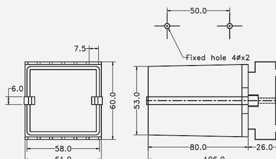
Outline dimension 外形尺寸
