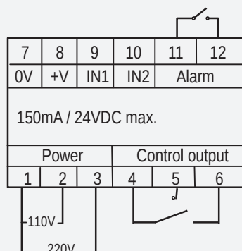
Connection diagram 接線圖
